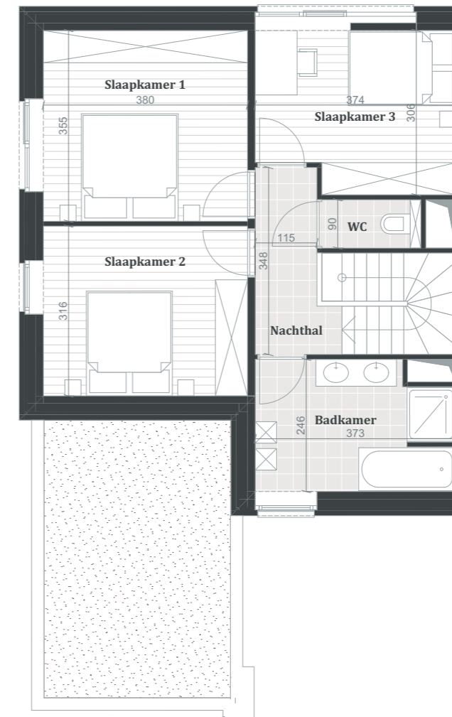
1e verdieping
