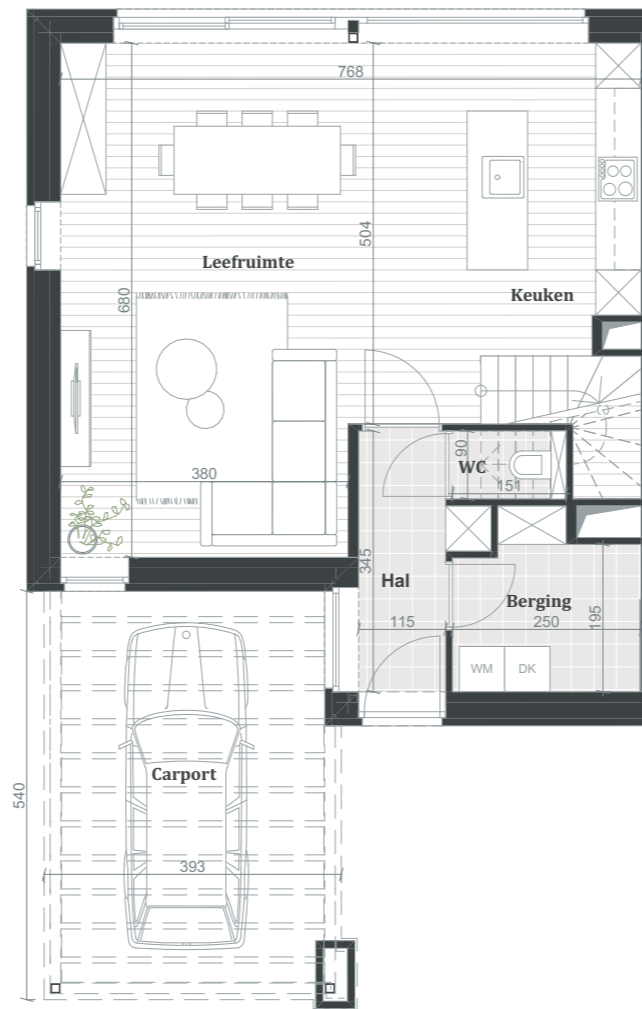
Gelijkvloers
